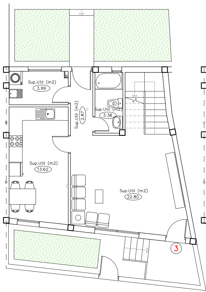
VIVIENDA 3 PLANTA BAJA
