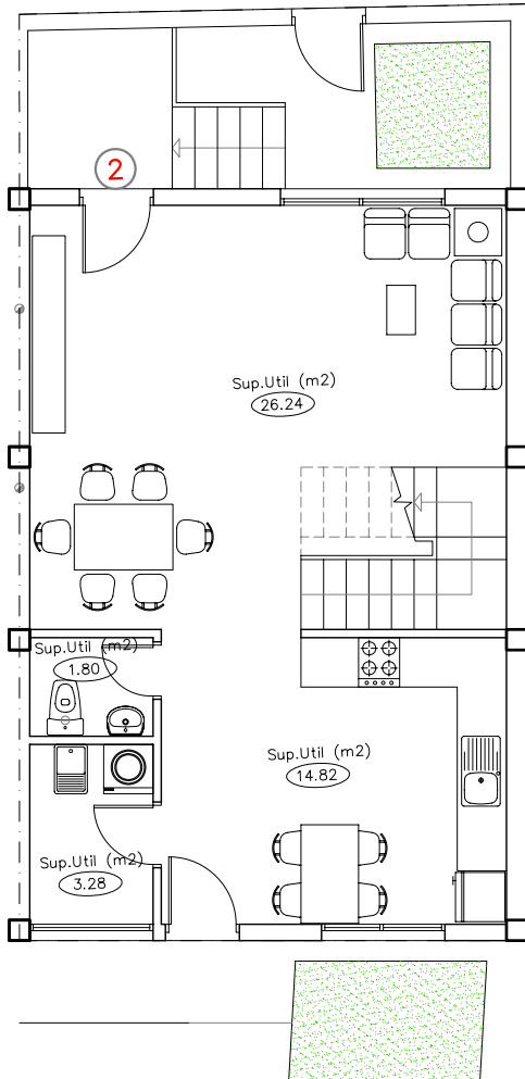
VIVIENDA 2 PLANTA BAJA
